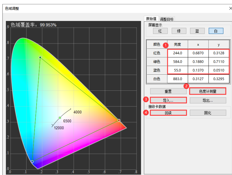
图 8.3.1 获取原始色域
