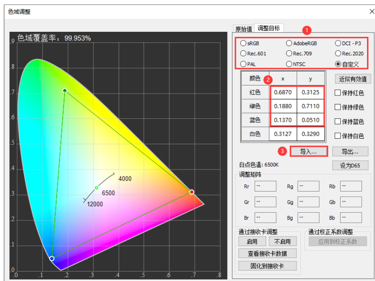
图 8.3.2 设置目标色域
