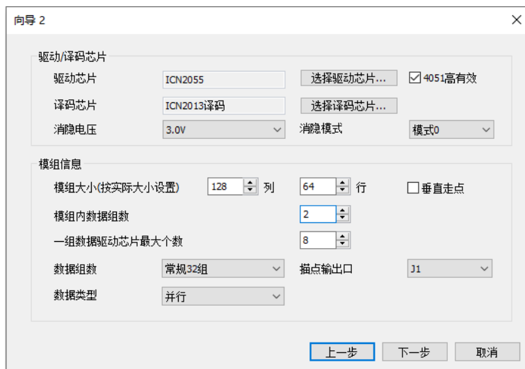
图 6.3.7.11 多类型模组向导 2
