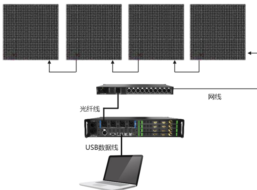
图 2.1.1 设备连接图
