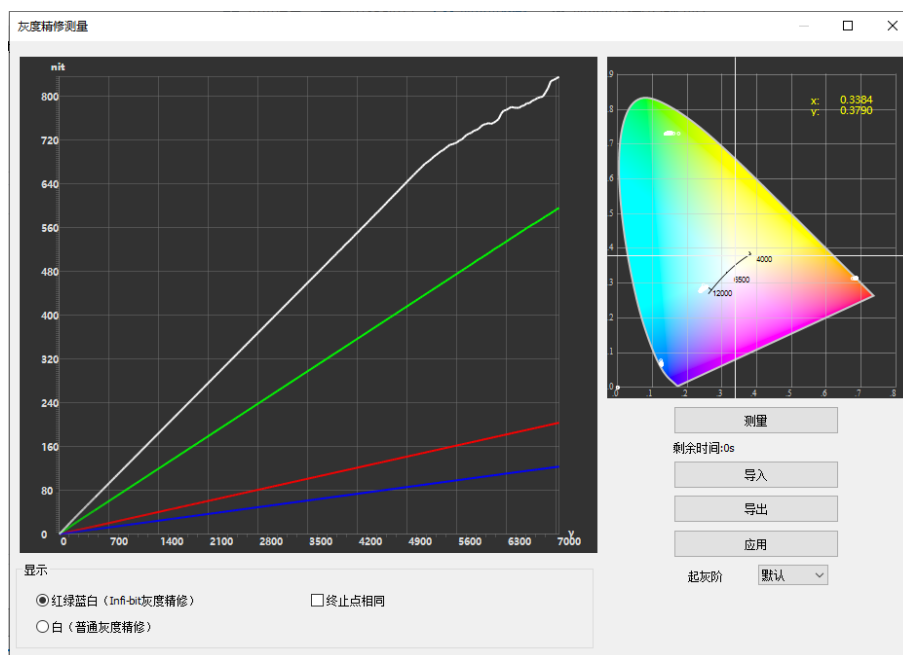
图 6.3.3.5 灰度精修测量
